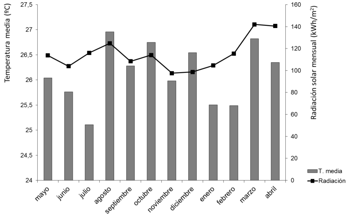
Figura 2. Temperatura media y radiación mensual registradas desde mayo 2015 a abril 2016. Santa Clara de San Carlos, Costa Rica.
