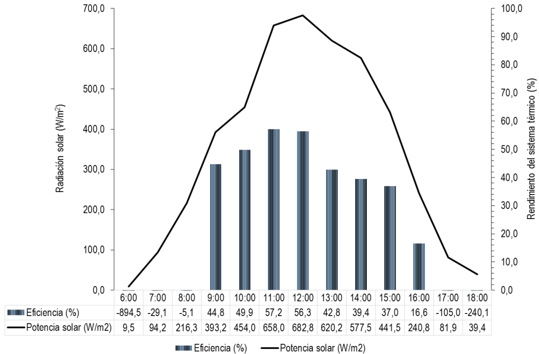
Figura 6. Rendimiento medio anual del sistema termosifónico a lo largo de un día, lechería del Instituto Tecnológico de Costa Rica, Sede Regional San Carlos (ITCR-SSC). Costa Rica.
