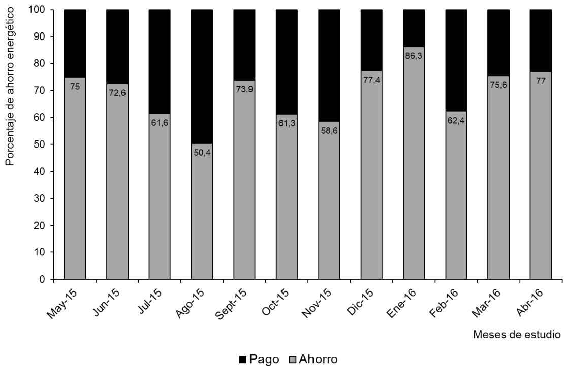
Figura 5. Ahorro energético porcentual logrado con el calentamiento del agua por medio del sistema termosifónico solar, de mayo de 2015 a abril 2016, lechería del Instituto Tecnológico de Costa Rica, Sede Regional San Carlos (ITCR-SSC). Costa Rica.
