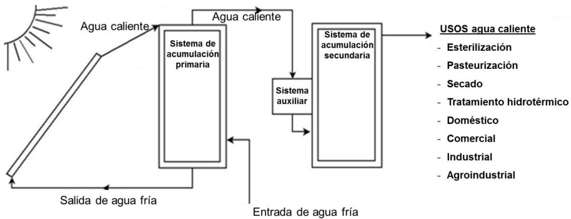
Figura 1. Esquema básico del sistema termosifónico híbrido instalado en la Lechería del Instituto Tecnológico de Costa Rica, Sede Regional San Carlos (ITCR-SSC), Costa Rica. 2015. El agua caliente asciende por diferencia de densidad hasta depositarse en el sistema de acumulación primaria. De su parte superior se canaliza a un segundo tanque que, junto con el sistema auxiliar, permite disponer de agua caliente a alta temperatura.
